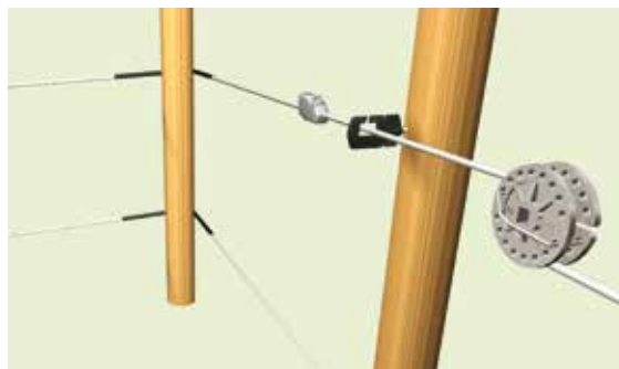
Bilde 19. Trådspstrammere gjør det enkelt å holde tråden stram.
